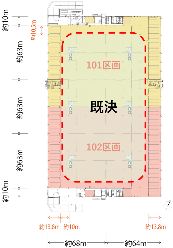
1 階平面図
