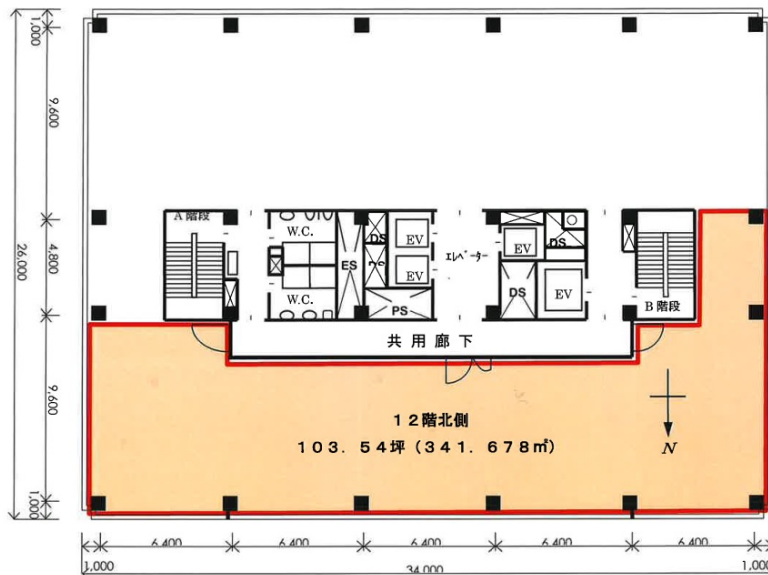
● 12階北側平面図
