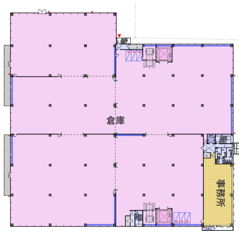
2階平面図
