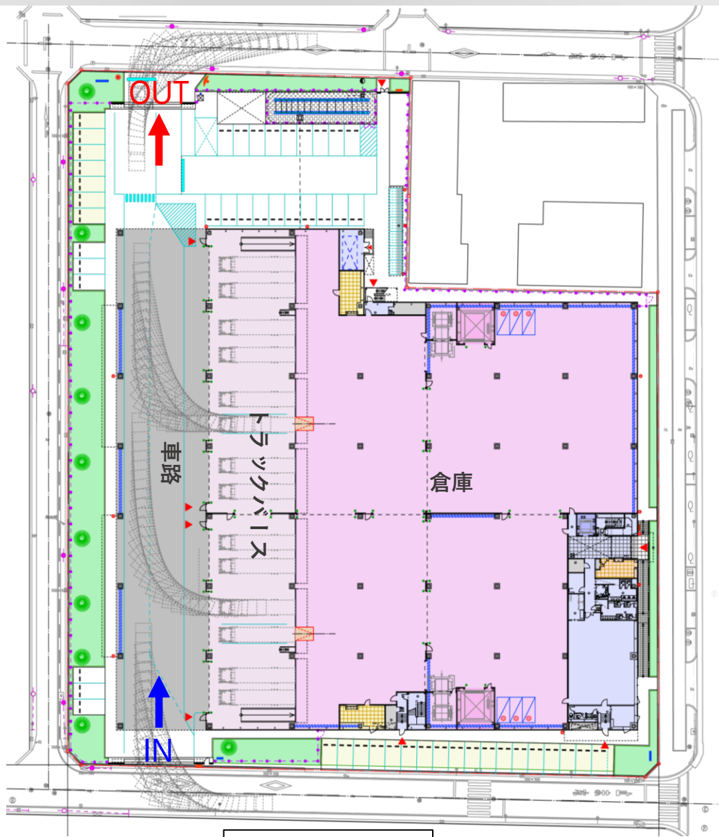
配置図兼1階平面図
