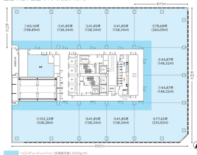
■基準階平面図 618坪(2,042㎡)
