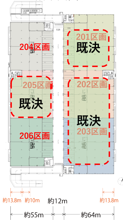
2階平面図
