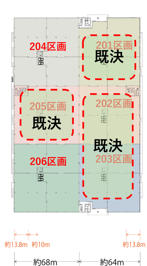
3階平面図
